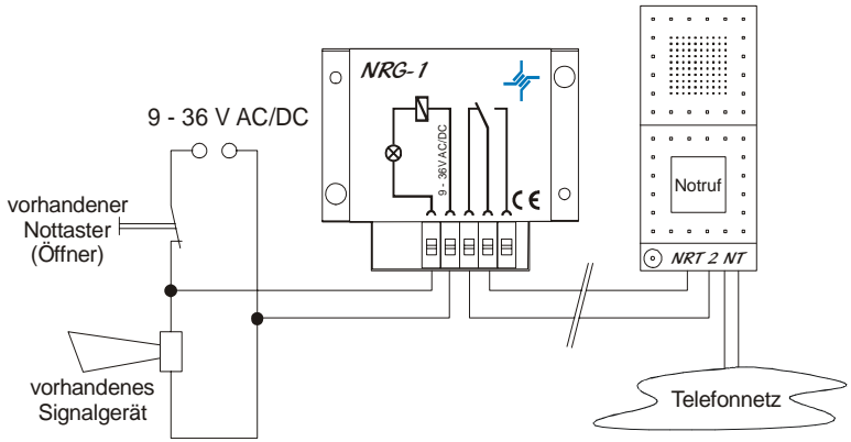
Vorhandener Nottaster ist Öffner, Notruftelefon NRT 2 NT braucht Schließer als Nottaste
