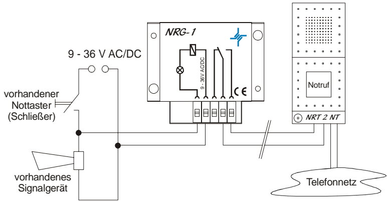
Vorhandener Nottaster ist Schließer, Notruftelefon NRT 2 NT braucht Schließer als Nottaste
